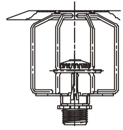
MODEL F1 UPRIGHT
