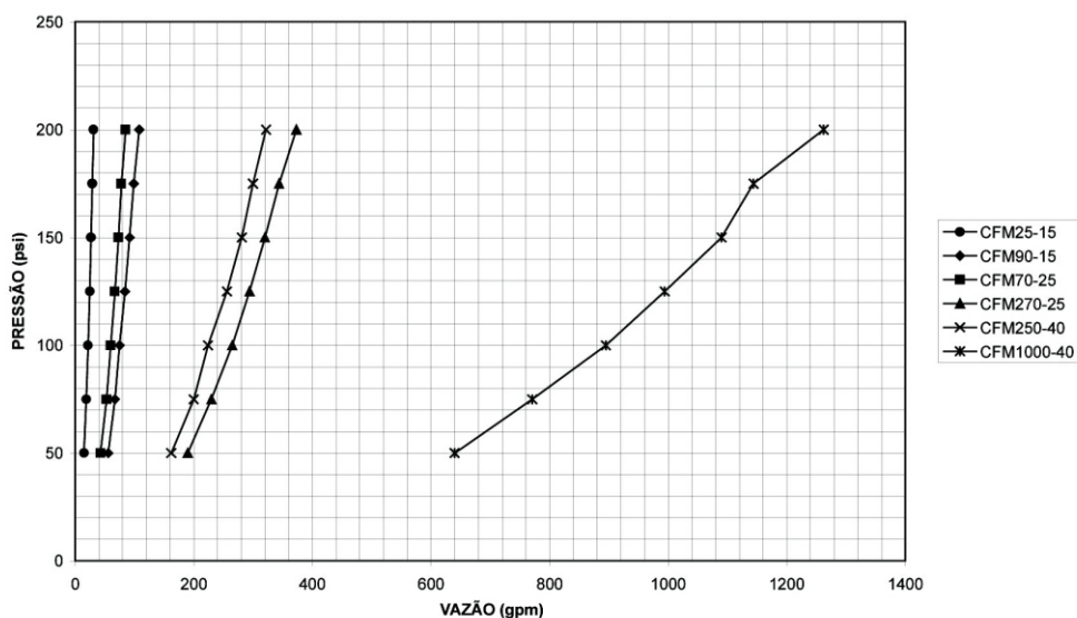
GERADOR DE ESPUMA DE ALTA CONTRAPRESSÃO DA CHEMGUARD VAZÃO X PRESSÃO
